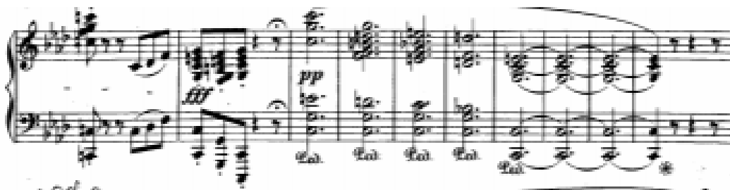
Slika 48- prikaz treće cjeline mosta prema codi četvrte balade u f-molu op.52
