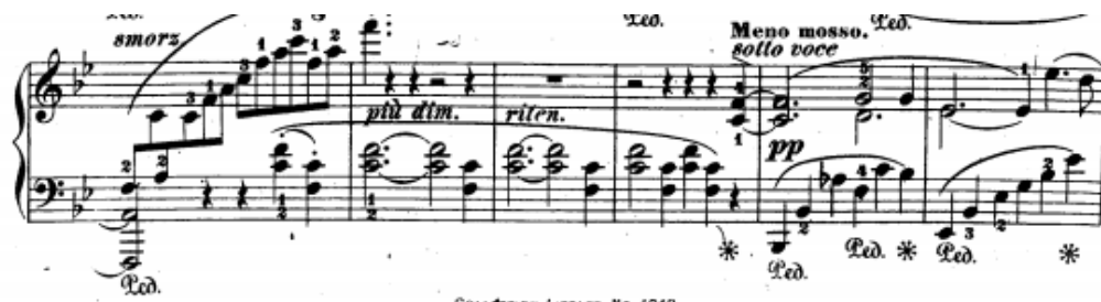
Slika 5- Druga tema prve balade u g-molu op.23 (takt 68)
