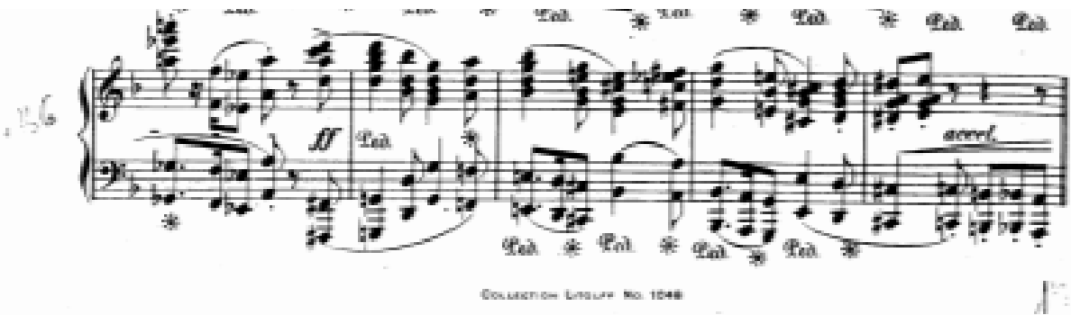
Slika 25- Završetak ponovljenoga Tempa I prve teme druge balade u F-duru op.38 ( takt 136-140)
