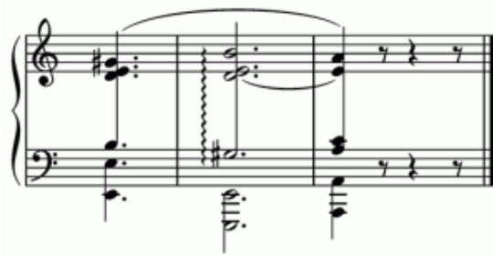
Slika 29 - prva verzija završetka druge balade u F-duru op.38
