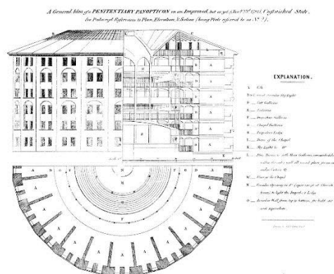
Slika 5 Nacrt konstrukcije zatvora po modelu panoptikona
