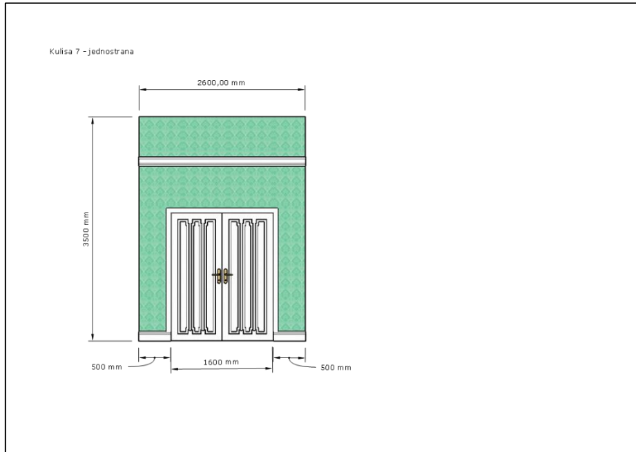
Slika 19. Tehnički nacrt unutrašnje kulise
