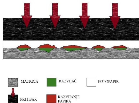
Prilog 16: Shema otiskivanja (razvijanja)
